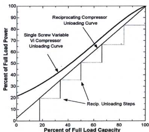
圖 9. 螺桿與往復式壓縮機部分負載與功耗之關係[5]
