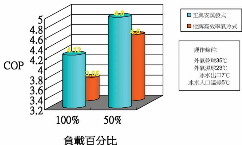
圖5.變負載效率比較
