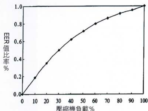
圖 10. 螺桿壓縮機部分負載時能效比的變化趨勢[6]
