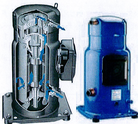
圖 2. Danfoss 公司 SY380 渦卷壓縮機 [ http://cn.drives.danfoss.com/ra/Products/ProductCatalogue.asp ]
