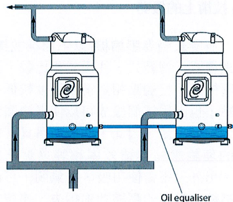
圖 5. 油氣平衡方式原理[3]
