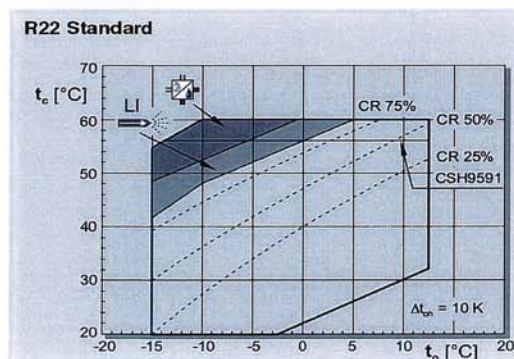
圖 11. 螺桿壓縮機應用範圍[5]
