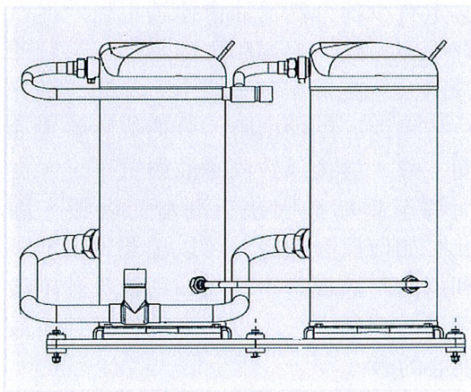
圖 4. 油氣平衡方式管線配置示意圖[3]
