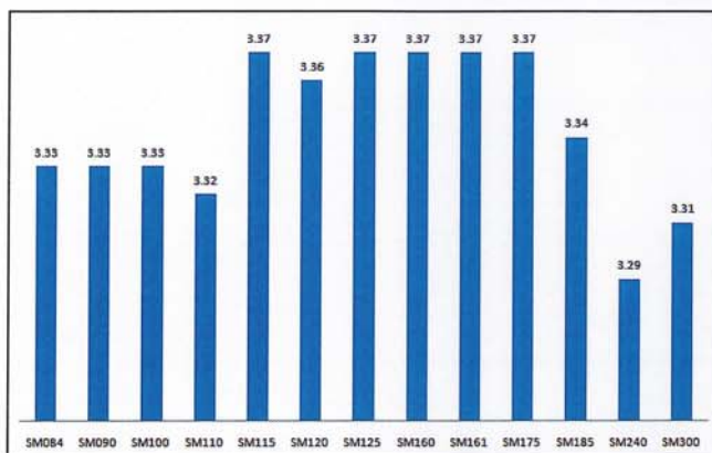
圖 7. Danfoss 公司 Performer 系列渦卷壓縮機單機能效比(COP)
