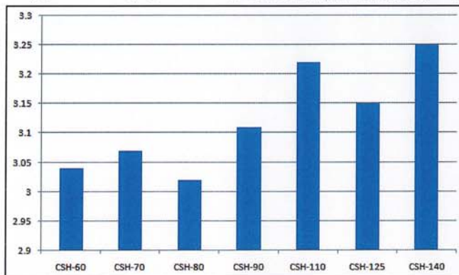
圖 8. Bitzer 公司 CSH 系列螺桿壓縮機單機能效比(COP)
