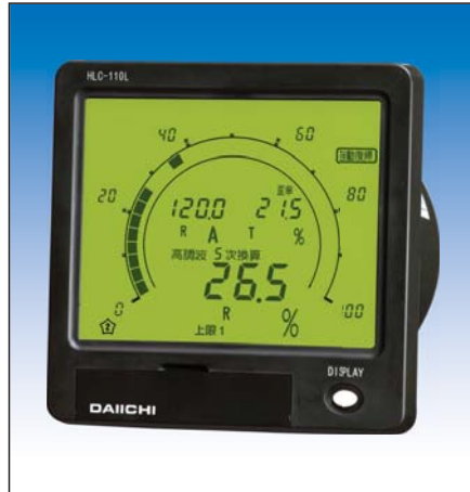
諧波測定器 HLC-110L HarmonicWave Meter HLC-110L
