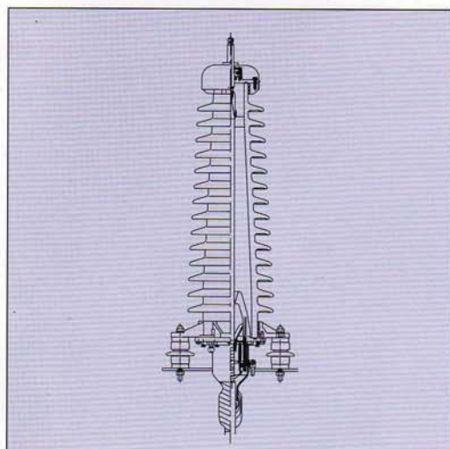
69KV 氣中電纜頭 69KV Cable Sealing End (EBA)
