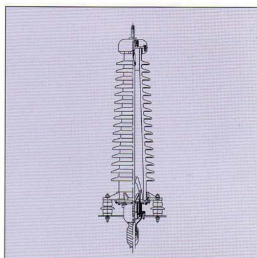
161KV 氣中電纜頭 161KV Cable Sealing End (EBA)
