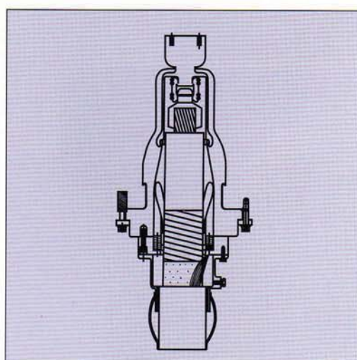
161KV SF6 氣封、油浸電纜頭 161KV (EBG(O)-S)
